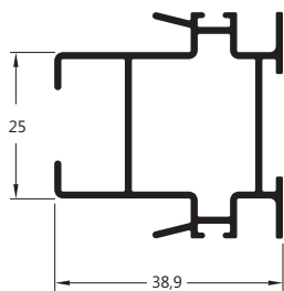
MG25-057 0,632 Kg/m Montante central intermediário sem baquete
