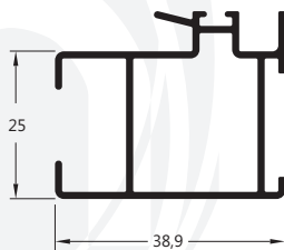
MG25-056 0,538 Kg/m Montante central sem baquete
