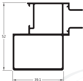
MG25-043 0,947 Kg/m Montante bi-tubular central da folha
