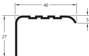
RA-013 0,268 Kg/m Remate
