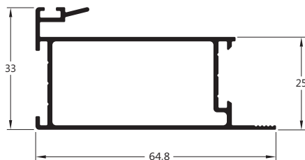
MG25-242 0,674 Kg/m Montante central externo da folha
