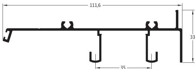
MG25-430 0,948 Kg/m Trilho intermediário integrada
