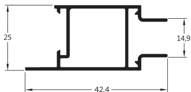
MG25-192 0,554 Kg/m Montante central da folha
