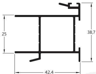
MG25-069 0,613 Kg/m Montante central intermediário veneziana
