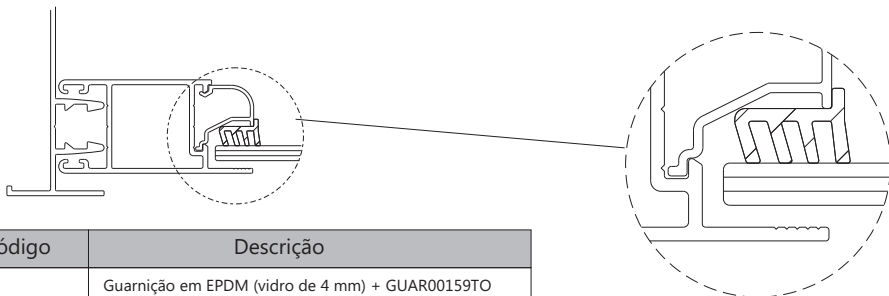
DETALHE DE APLICAÇÃO sem escala
