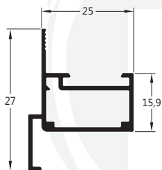
MG25-097 0,399 Kg/m Montante báscula
