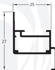
MG25-098 0,399 Kg/m Montante báscula
